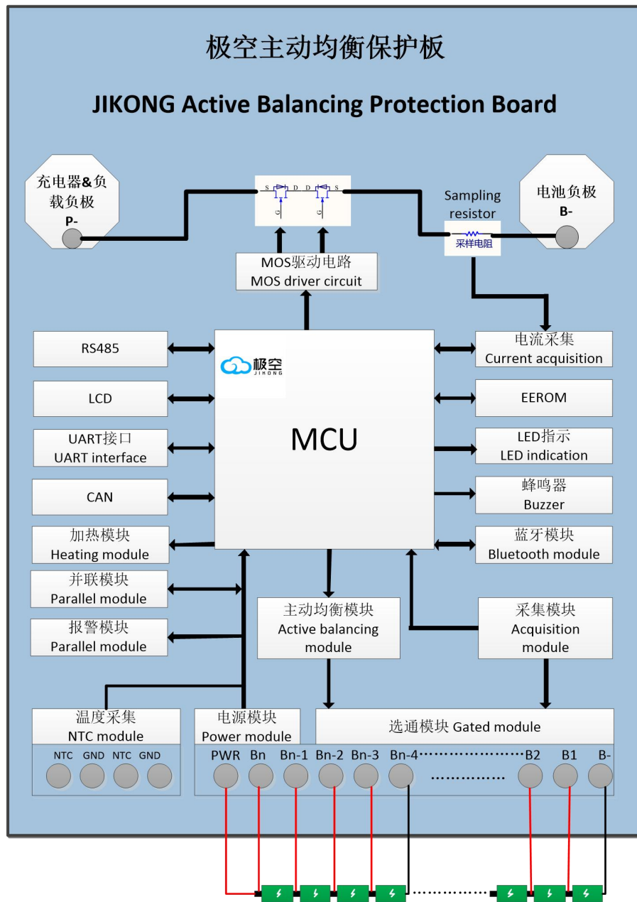
JK-B1A8S-10PS 结构框图
