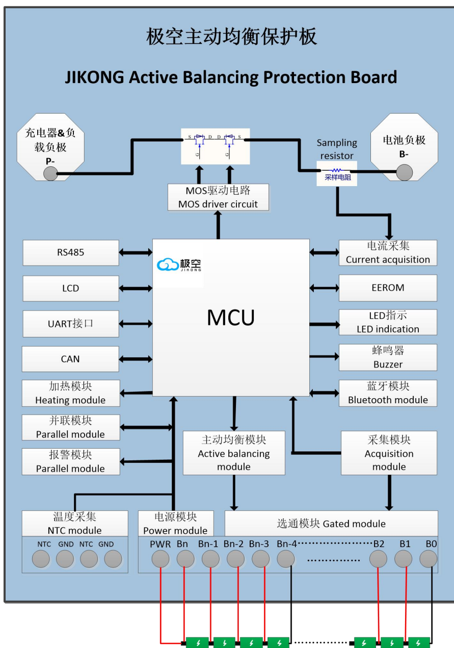
JK-BD4AxxS-12P 结构框图
