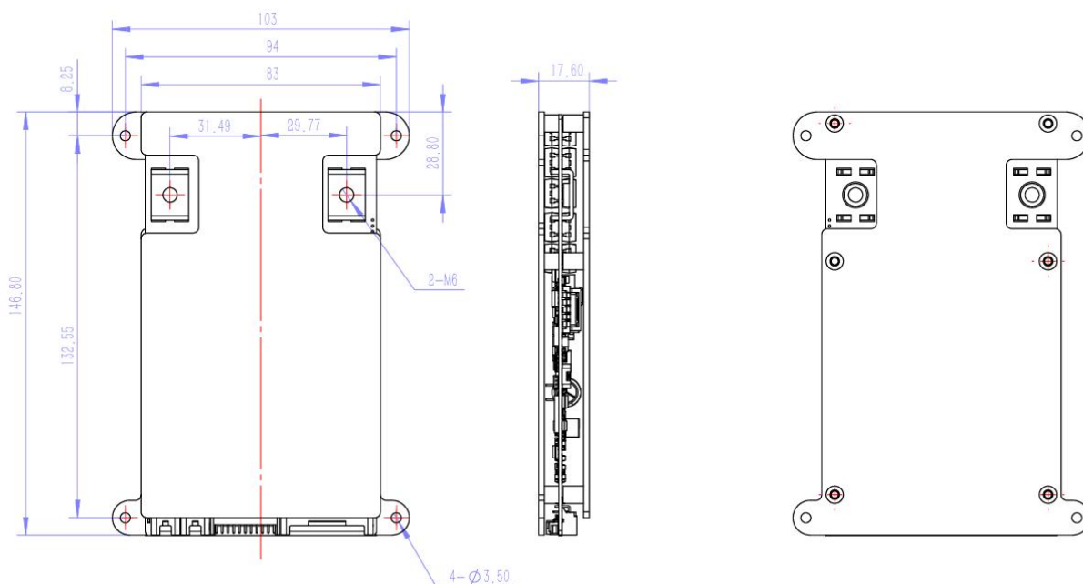
JK-BD4AxxS-12P外形尺寸
