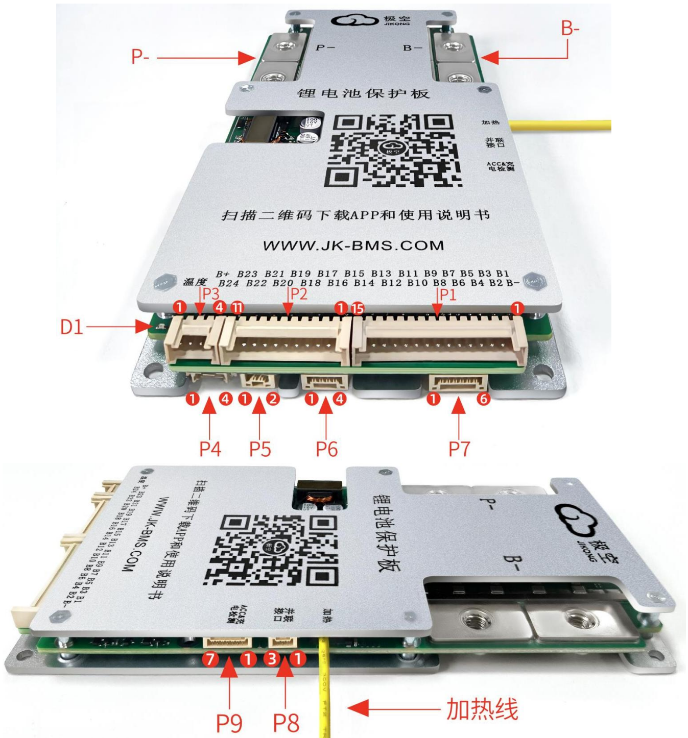
JK-BD6A24S-15PD连接器示意图
