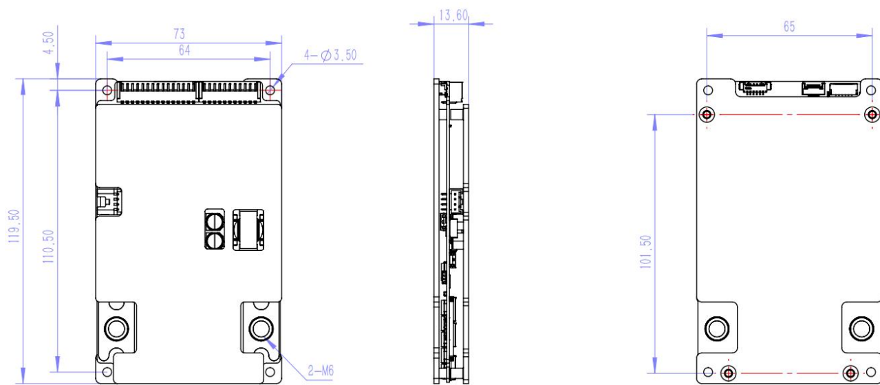
JK-BD6A24S-4PD 外形尺寸
