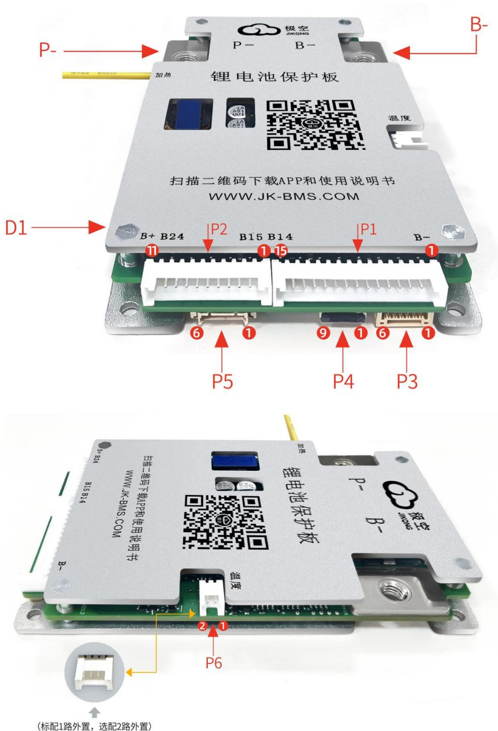
JK-BD6A24S-4PD 连接器示意图
