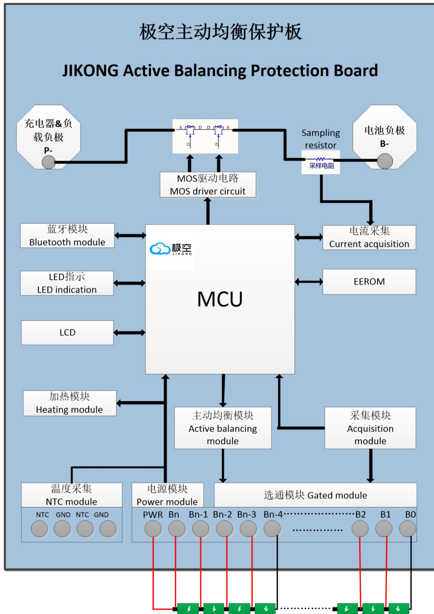
JK-BD6A24S-4PD 结构框图
