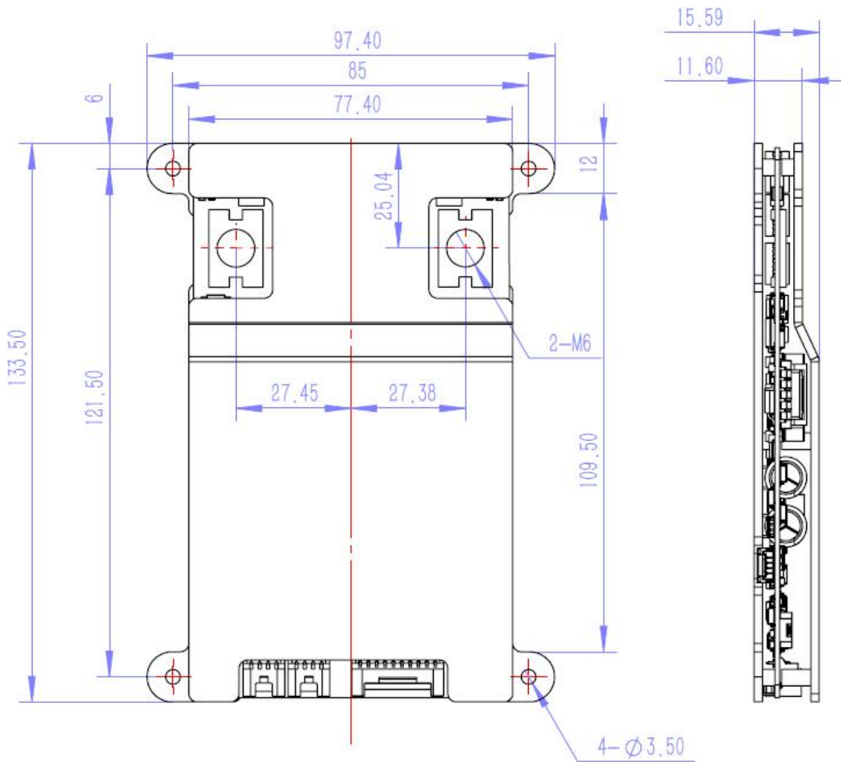
JK-BD6A8S-10P 外形尺寸
