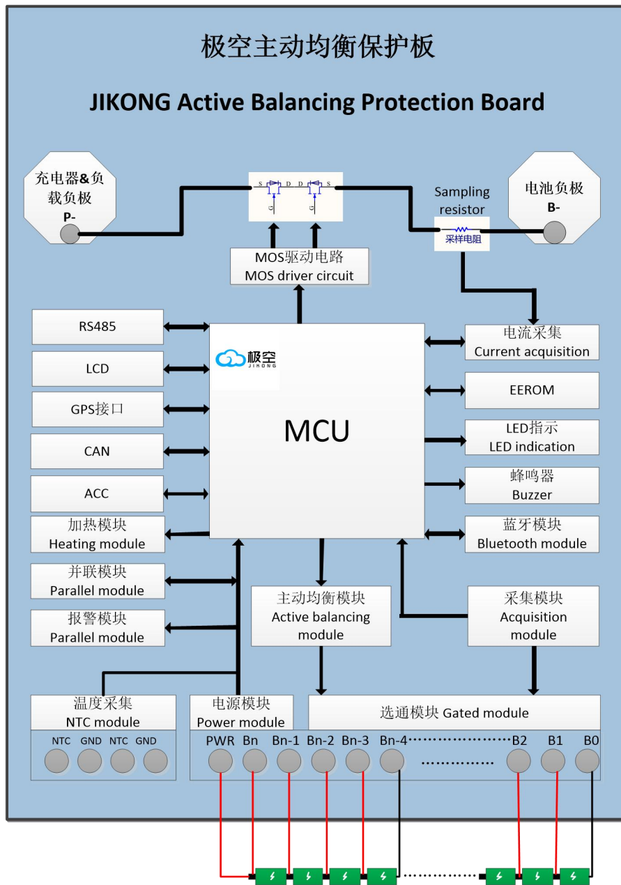
JK-BD6A8S-10P 结构框图
