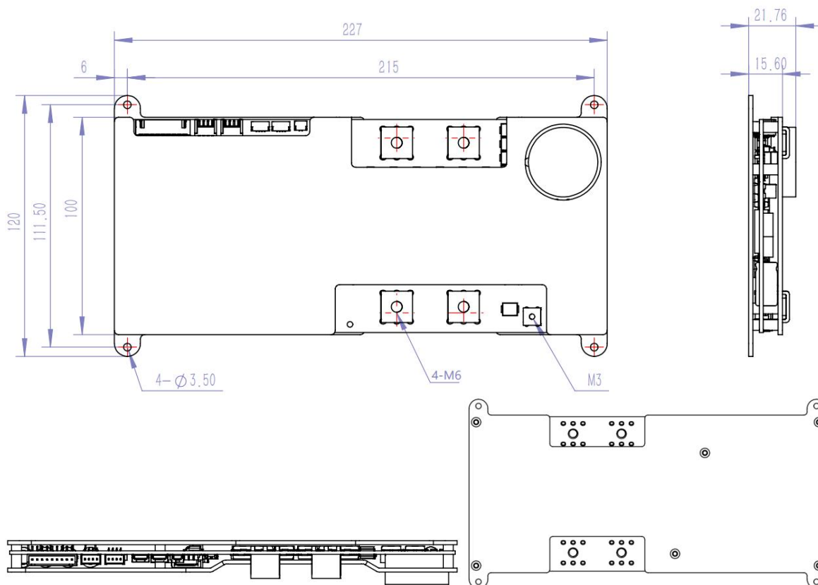
JK-QB2A8S-20P 外形尺寸
